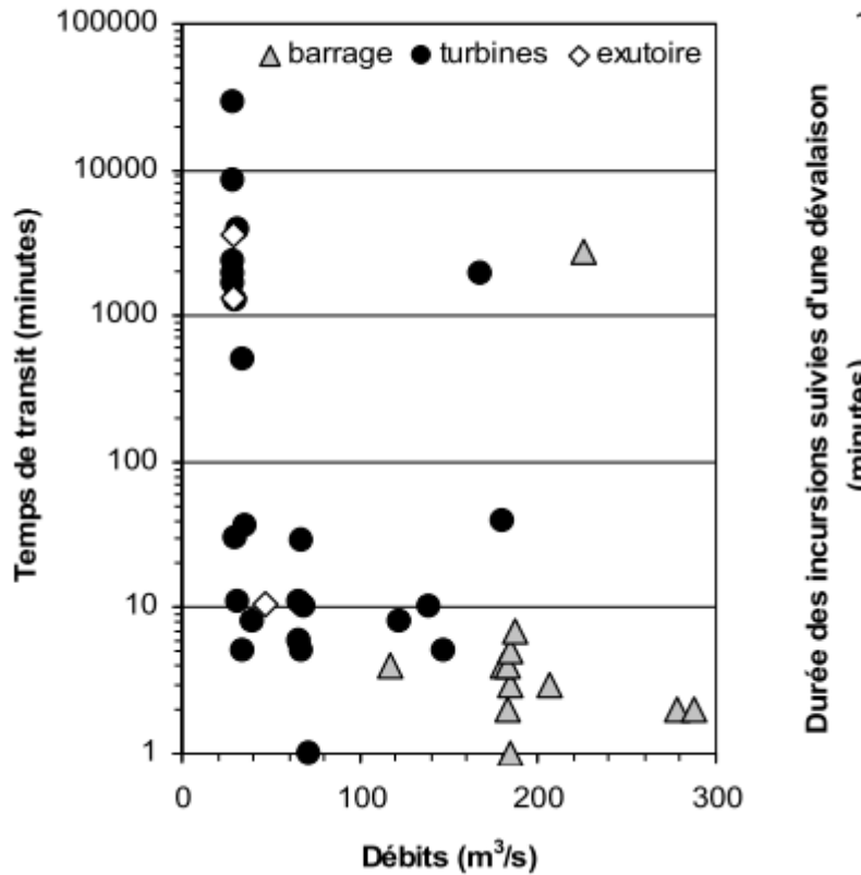
Dans : [TRAVADE 2008] Figure 3.14 : Variabilité des temps de transit et de dévalaison suivant les débits du Gave au moment des passages à Artix par les différentes voies
