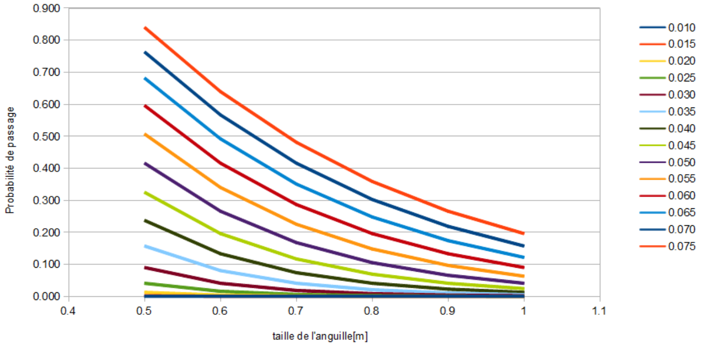
Probabilité de passage de grille pour différents espacements [m]
